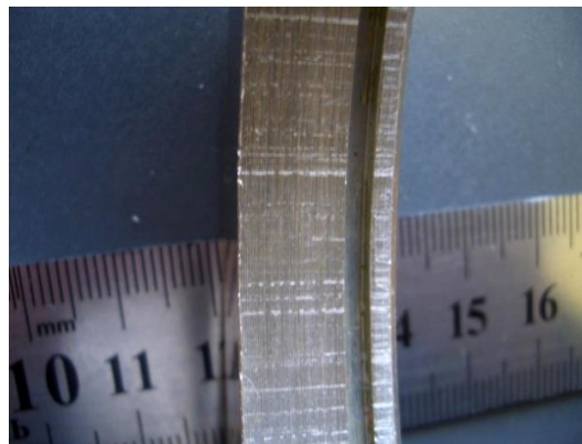
Рис. 7. Участок модельного образца с дефектами в виде поверхностных трещин после полива флюоресцентной магнитной суспензией. Облучение ультрафиолетовой лампой
