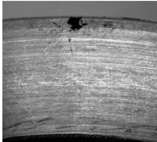
Рис. 4. Язвенная коррозия кольцевого образца из стали 09X16N4Б-Ш после вылеживания в 25 %-ном растворе морской соли при комнатной температуре
