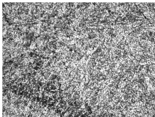
Рис. 1. Микроструктура стали 09X16H4Б-Ш, ×1000
