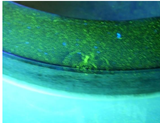
Рис. 6. Участок модельного образца с язвенной коррозией вблизи внешней цилиндрической поверхности после полива флюоресцентной магнитной суспензией. Облучение ультрафиолетовой лампой
