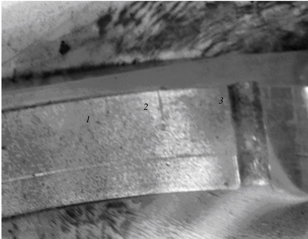
Рис. 8. Результаты измерения тангенциальной составляющей вектора магнитной индукции на поверхности образца после испытаний на коррозию под напряжением
