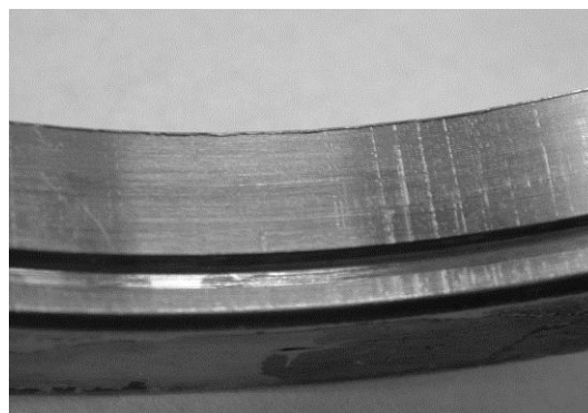
Рис. 5. Дефекты на внутренней поверхности кольцевого образца из стали 09X16N4Б-Ш после вылеживания в 25 %-ном растворе морской соли при комнатной температуре в течение 6 мес 12 дней
