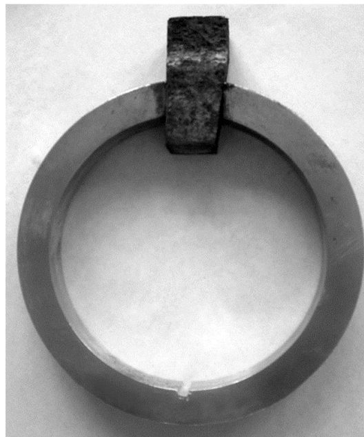
Рис. 3. Внешний вид кольцевого образца, подвергаемого испытанию на коррозию под напряжением
